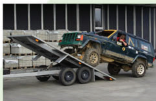
Přívěsný vozík sklopný plošinový 3038-5860-294-9436 délka podlahy 4 000 mm
